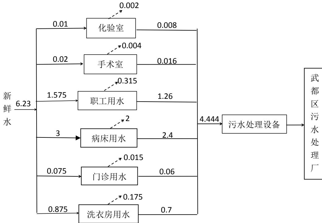
图 2-3 本项目运营期水平衡图 单位: m 3 /d
