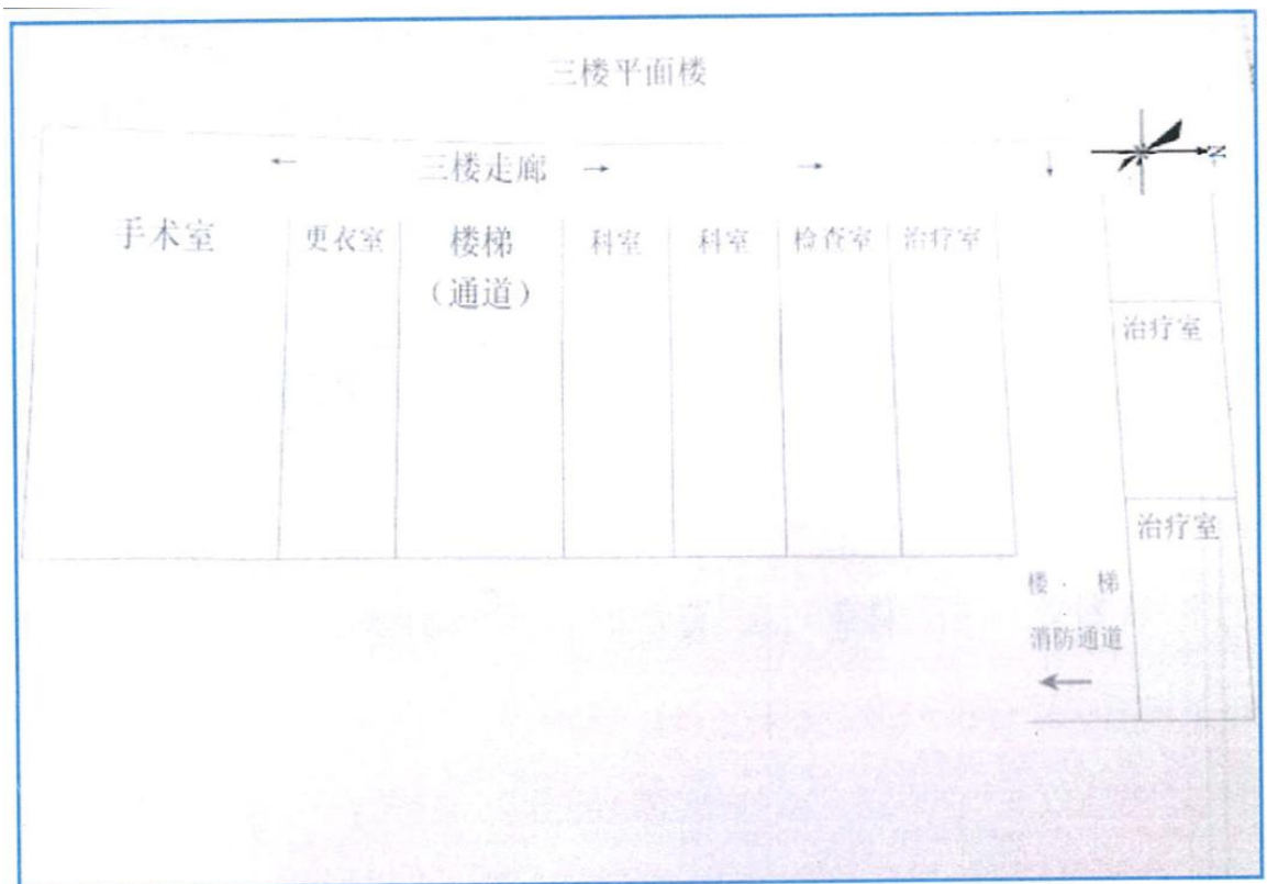
图 2-2 (3) 三层平面布置图
